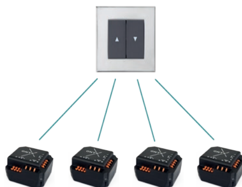
Variante 2: Gruppensteuerung kabelgebunden
